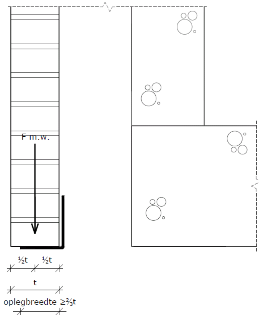
Figuur 4 - Positie belasting op lateien zonder/met onvoldoende spouwankers
