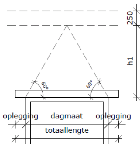
Figuur B1 – Aannames belasting op lateien (schematisch weergegeven)
