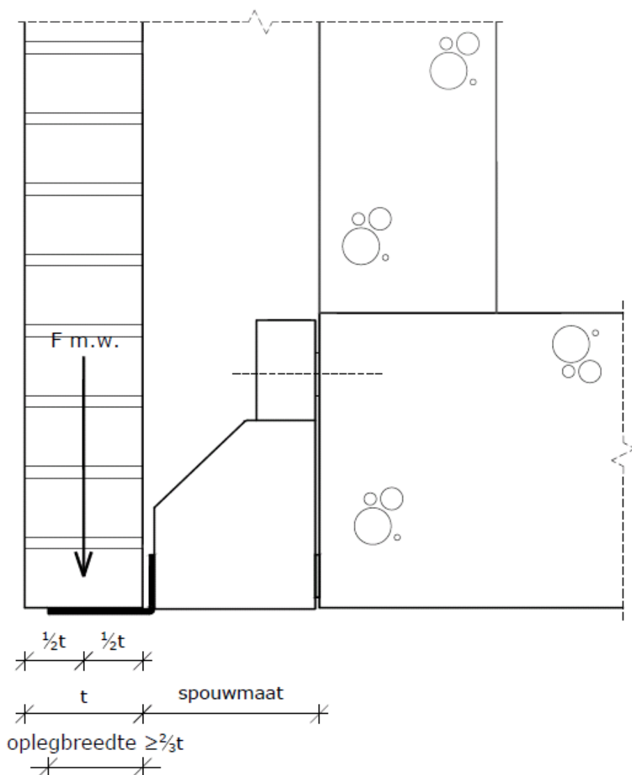
Figuur 2 - Positie belasting op metselwerkondersteuning zonder/met onvoldoende spouwankers
