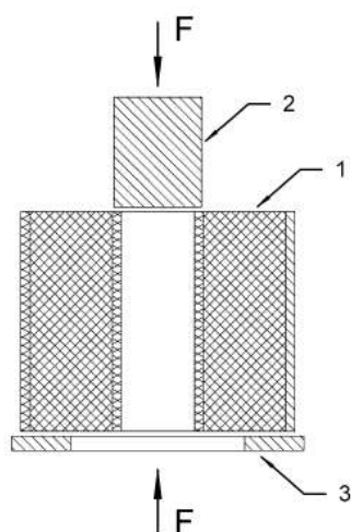
Figuur 11-2 Beproeblingsapparaat afschuifsterkte
