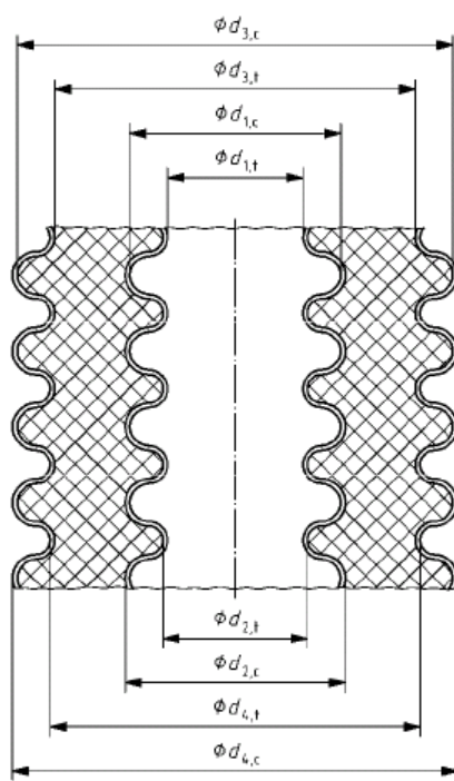
Figuur 17-2 Diameters van geribbelde buis
