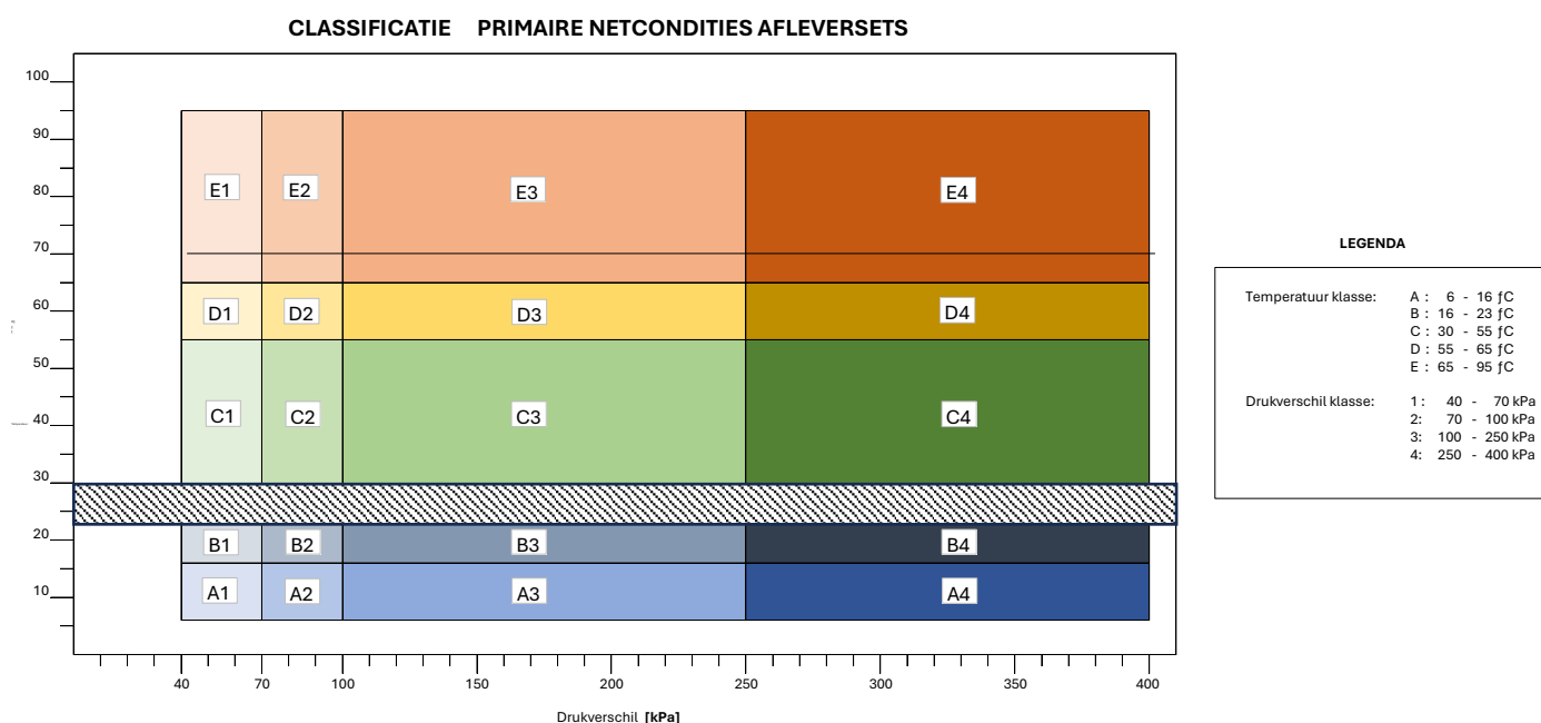
Figuur 2: Netklasse - classificatie van primaire netcondities
