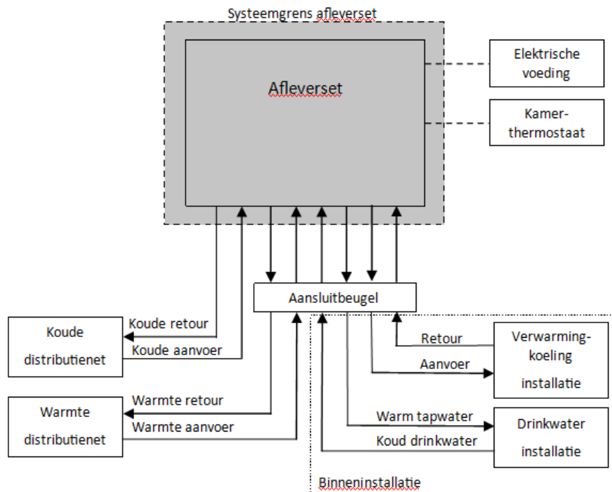
Figuur 1: Voorbeeld van de systeemgrenzen en interfaces van de afleverset
