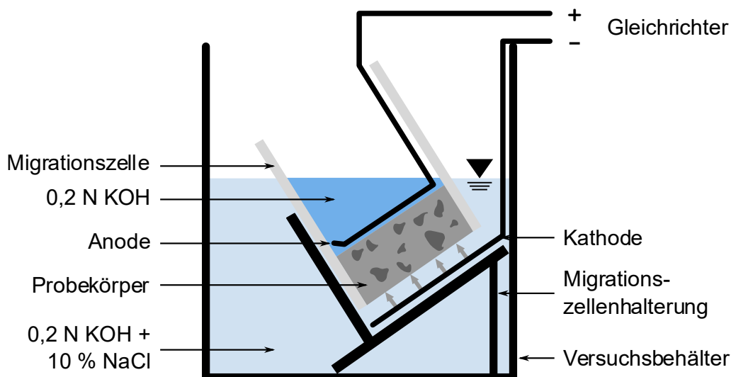
Abbildung 5 Schematische Darstellung des Messaufbaus (entnommen aus der Arbeitsanweisung Schnellbestimmung von Chloriddiffusionskoeffizienten für Betonprüfkörper, ibac) und Foto der Messzelle mit Netzteil und Verteilerbox
