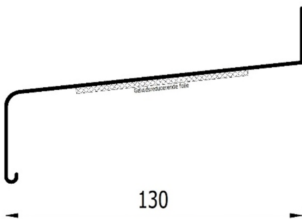
Figuur 3 – Waterslagen Euro Aluminium 58000 serie
