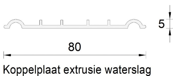
Figuur 5 – Koppelplaat extrusie waterslag
