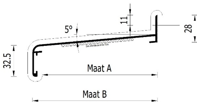
Figuur 2 – Waterslagen Euro Aluminium 56000 serie
