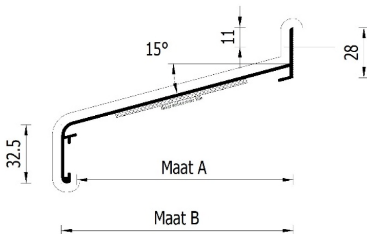
Figuur 1 – Waterslagen Euro Aluminium 54000 serie
