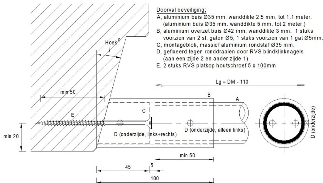
Figuur 2 – Doorvalbeveiliging, optie 2a/2b
