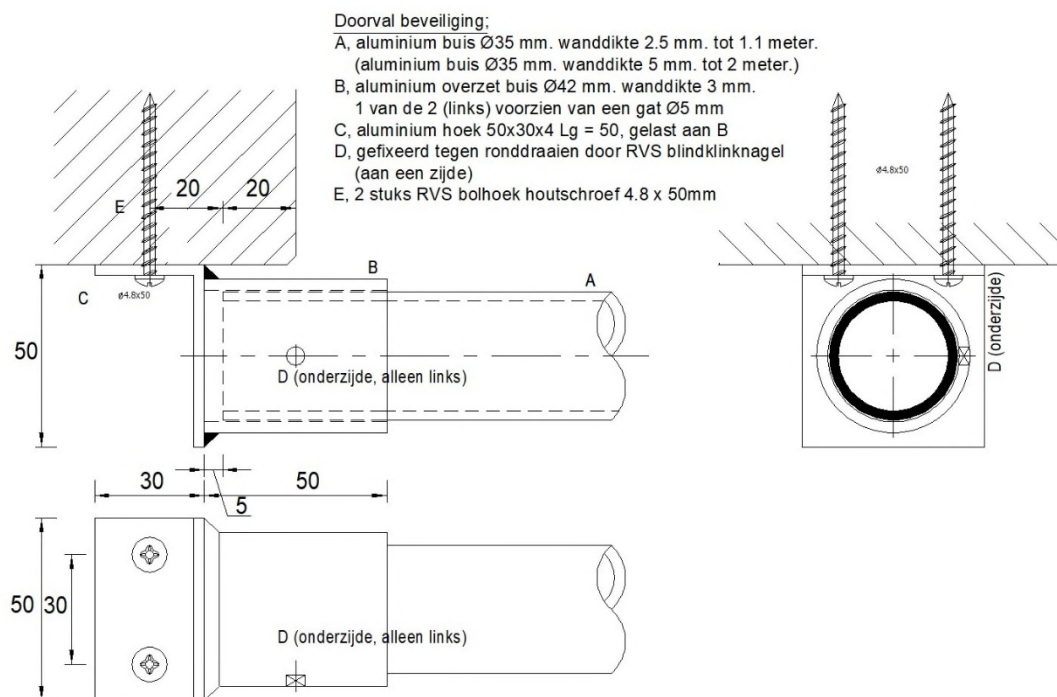
Figuur 3 – Doorvalbeveiliging, optie 3a/3b
