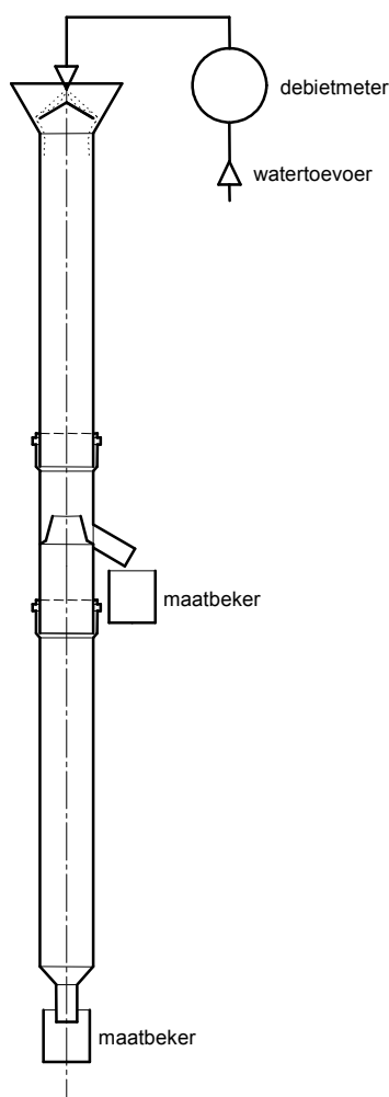
Figuur 9: Beproevingsofstelling voor testen van een condensafscheider
