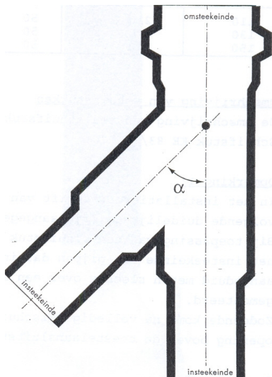
Figuur 5: T-stuk met insteekteinden en omsteekteinde
