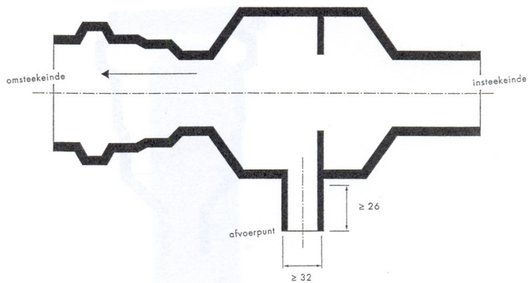
Figuur 7: Condensafscheider voor horizontale plaatsing met insteekende en omsteekende. Maten in mm. ( \varnothing 32 mm omvat de uitwendige diameter)
