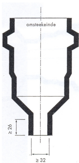
Figuur 8: Condensopvanghulpstuk met omsteekende. Maten in mm. ( \varnothing 32 mm omvat de uitwendige diameter)
