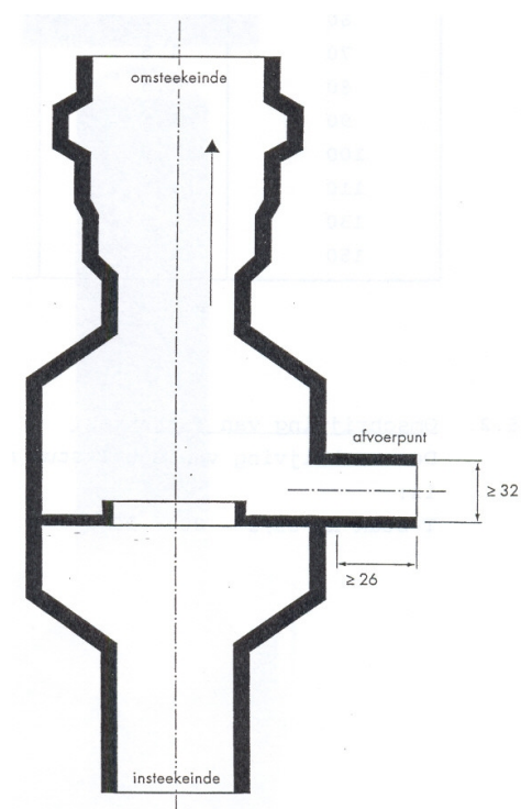
Figuur 6: Condensafscheider voor verticale plaatsing met insteekende en omsteekende. Maten in mm (Ø 32 mm omvat de uitwendige diameter)
