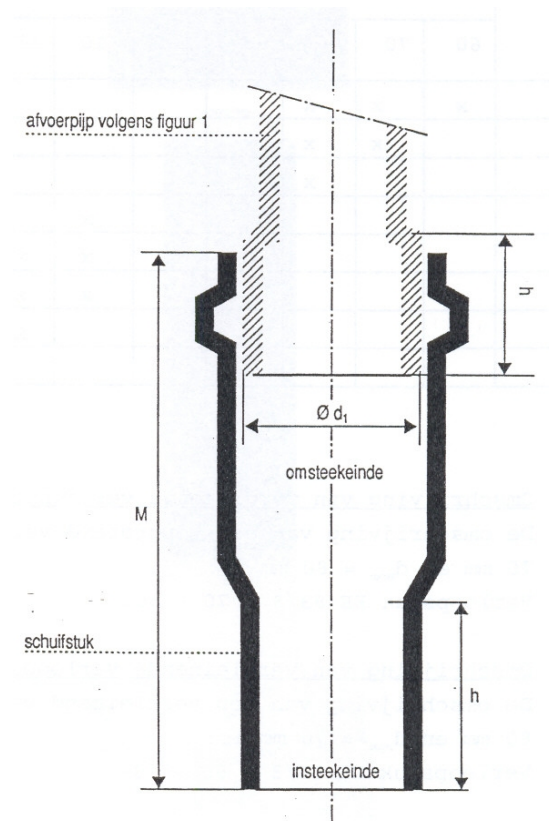
Figuur 4. Schuifstuk met insteekende en omsteekende
