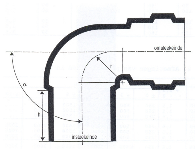
Figuur 2: Bocht met insteekkeinde en omsteekkeinde
