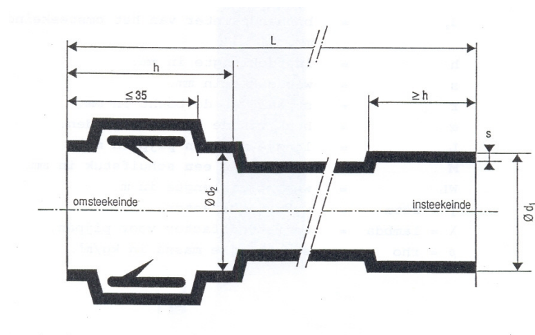
Figuur 1: Pijp met insteekteinde en omsteekteinde
