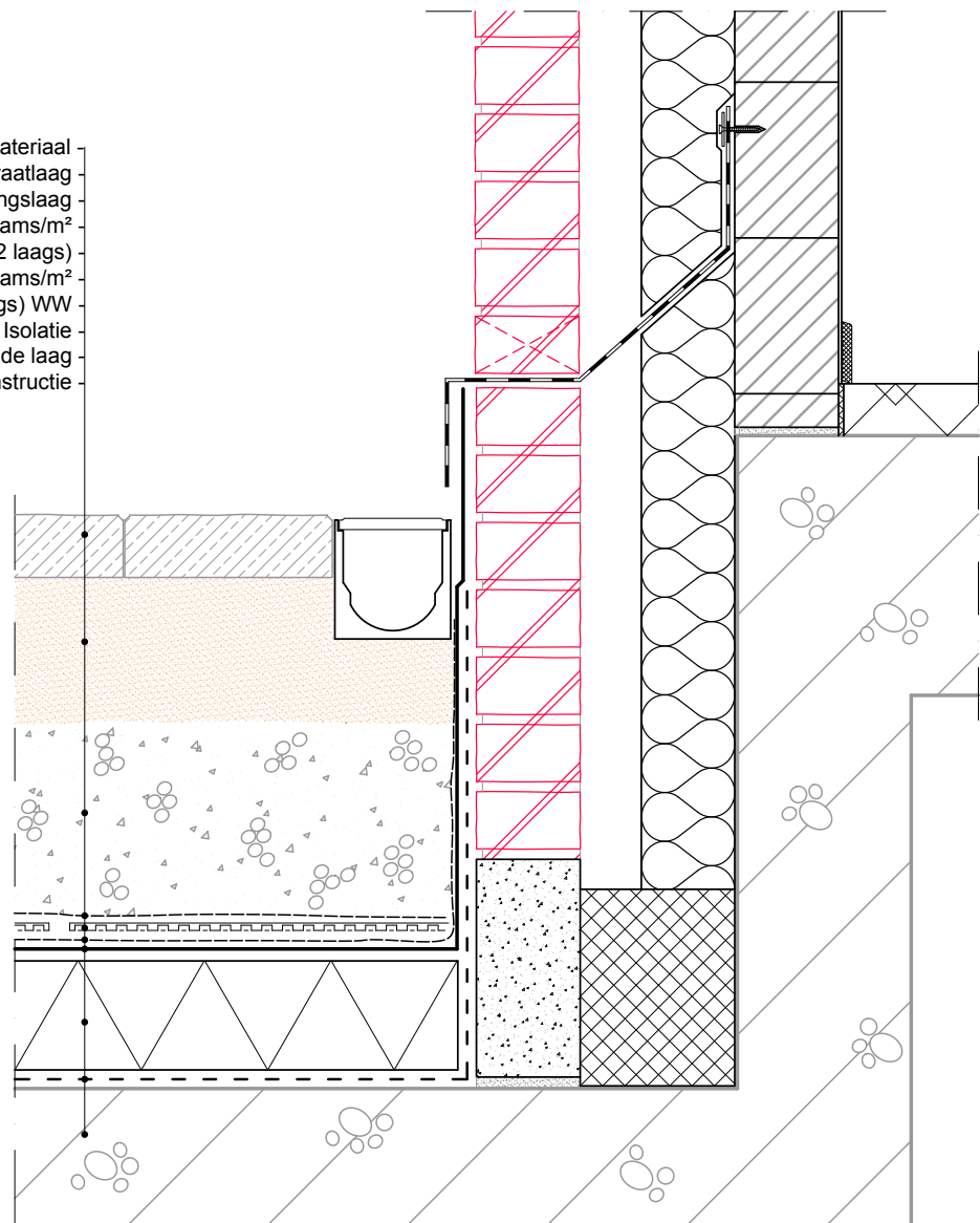
Dakinrichting Rijverharding
