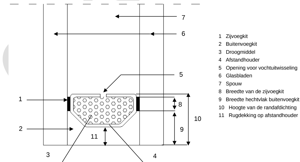
Figuur 1 - Systeem van een tweevoudige randafdichting
